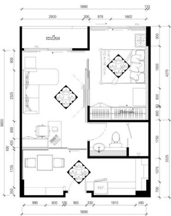
แปลนเฟอร์นิเจอร์ SCALE 1:50
